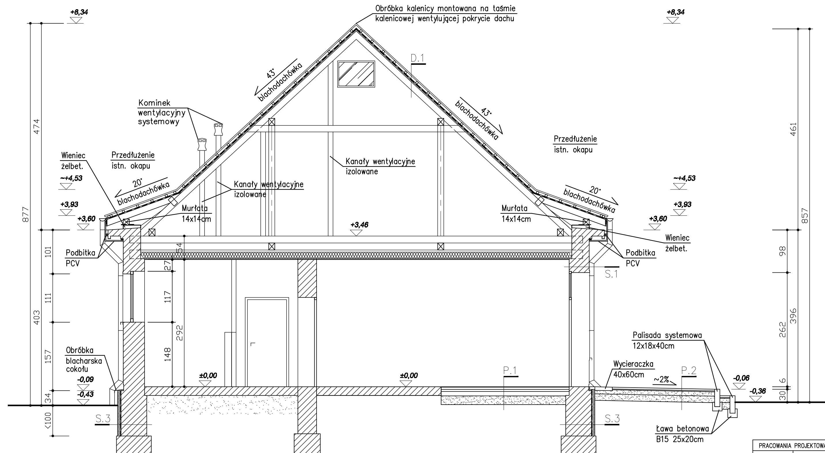
PRZEKRÓJ 2-2
